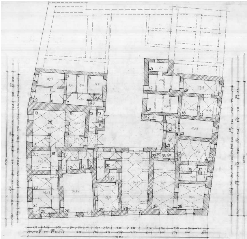
Zoisova palača, tloris pritličja, vir: ZVKDS, M. Stražišar, 1982
