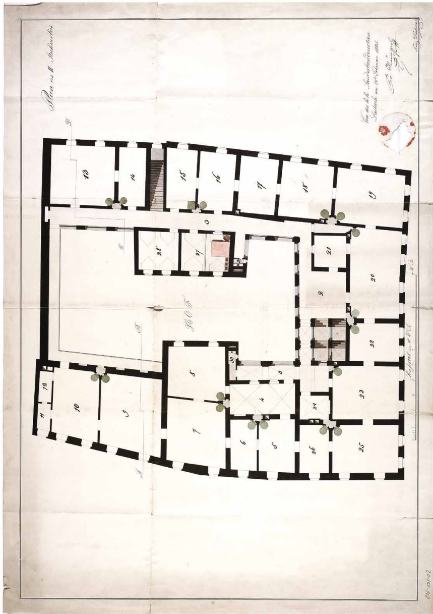
24. Franc Dežman, Tloris druga nadstropja palače, 1825, SI ZAL, Zbirka načrtov, 334-016-001-002
